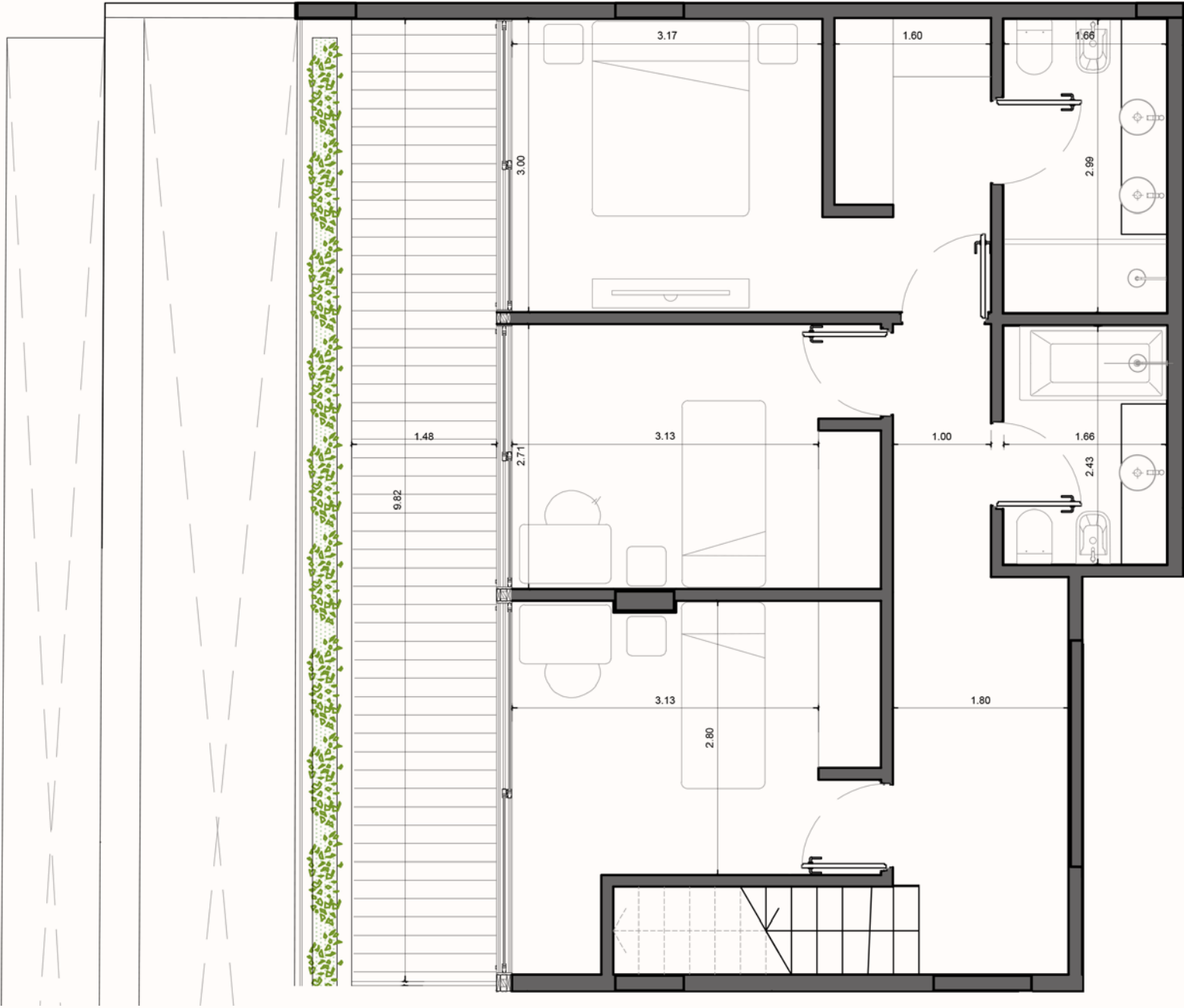
PLANTA BAJA
